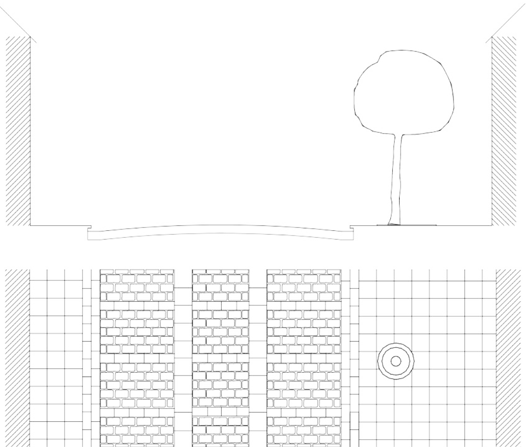
Tipo B2. Conci irregolari di pietra, disposti a riquadri, incorniciati da conci regolari, con compluvi laterali in pietra. Marciapiedi a formelle quadrate in pietra. Dal lato più largo presenza di fogliame di medio fusto.
