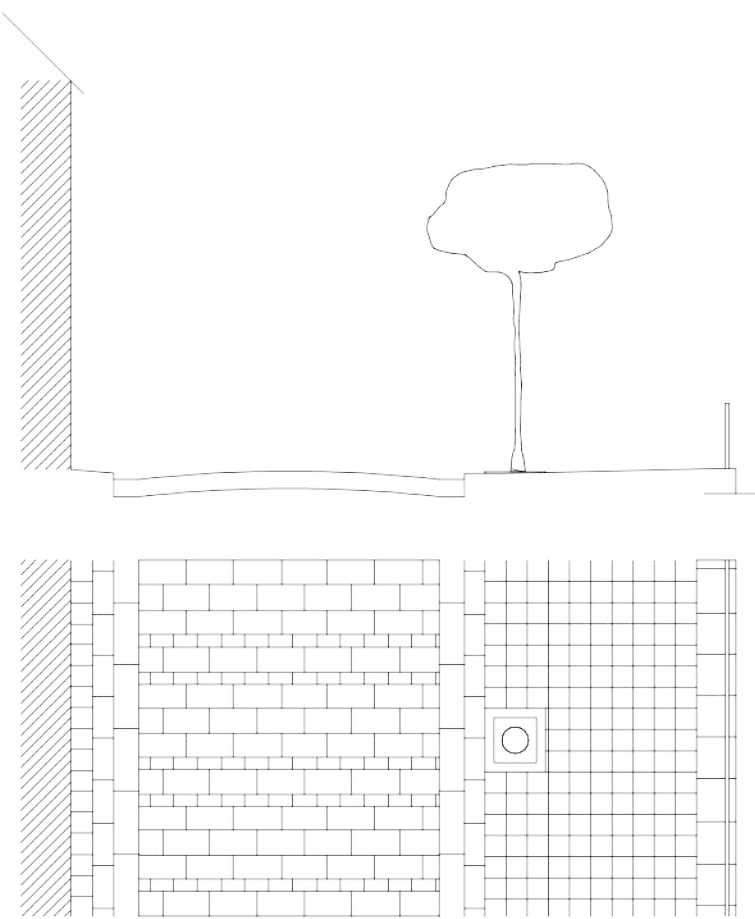
Tipo C5. Basole in pietra di forma regolare con assestamento a fasce di dimensioni diverse. Compluvi laterali in pietra. Marciapiedi lastricati con basole in pietra di forma quadrata.
