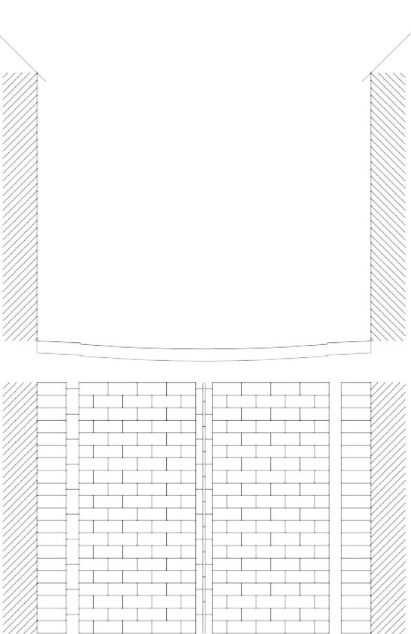
Tipo A4. Piano stradale in pietra, compluvio centrale. Marciapiede in pietra con gradino raccordato.
