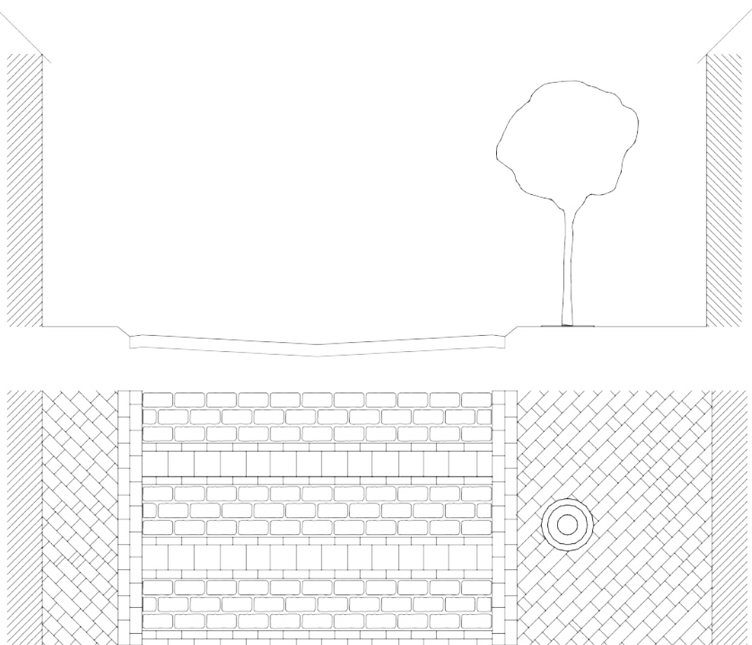
Tipo B3. Conci di pietra di forma regolare alternati a conci di pietra di forma irregolare, disposti a fascia. Compluvio centrale. Marciapiede raccordato al piano stradale con conci di forma regolare, lastricato con formelle di pietra.
