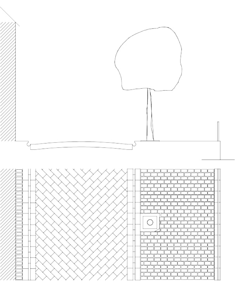
Tipo C3. Basole in pietra disposte a spina di pesce. Compluvi laterali in pietra. Marciapiedi in conci irregolari di pietra e dentello a conci in pietra di forma regolare.
