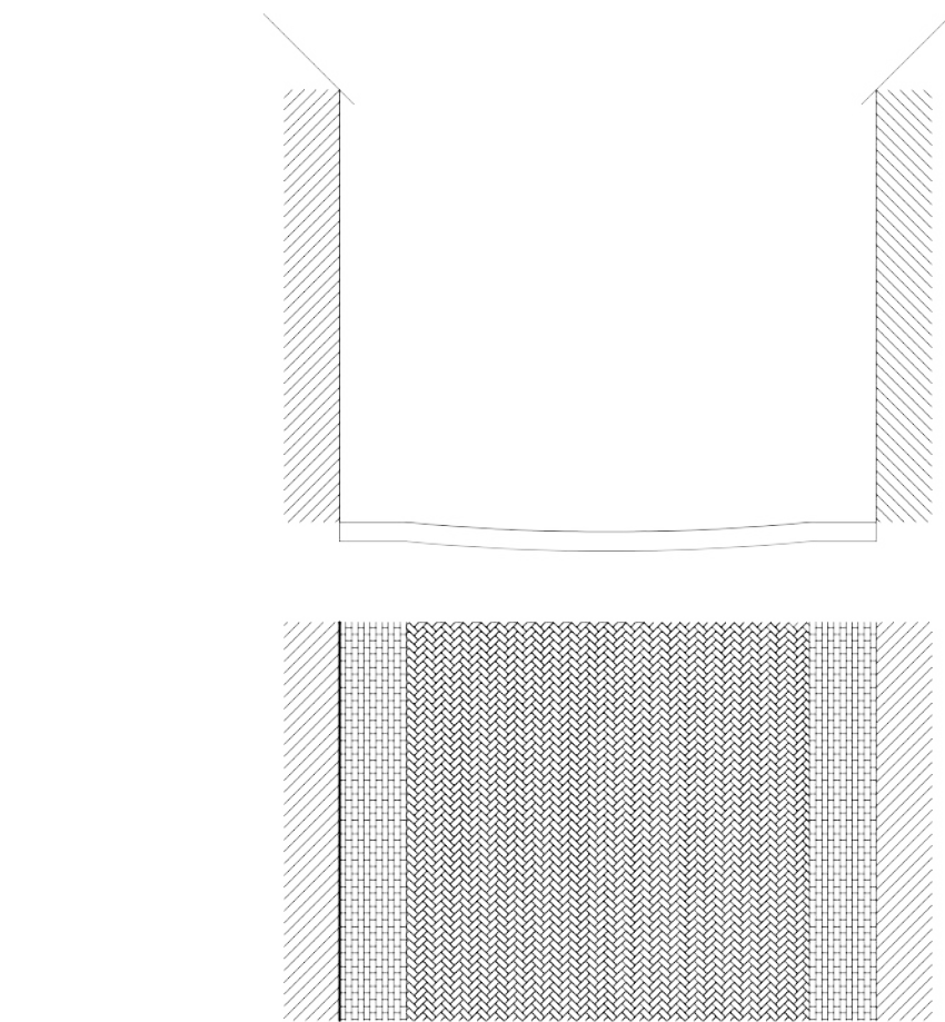
Tipo A1. Pavimentazione in mattonelle di pietra o asfalto con compluvio centrale.
