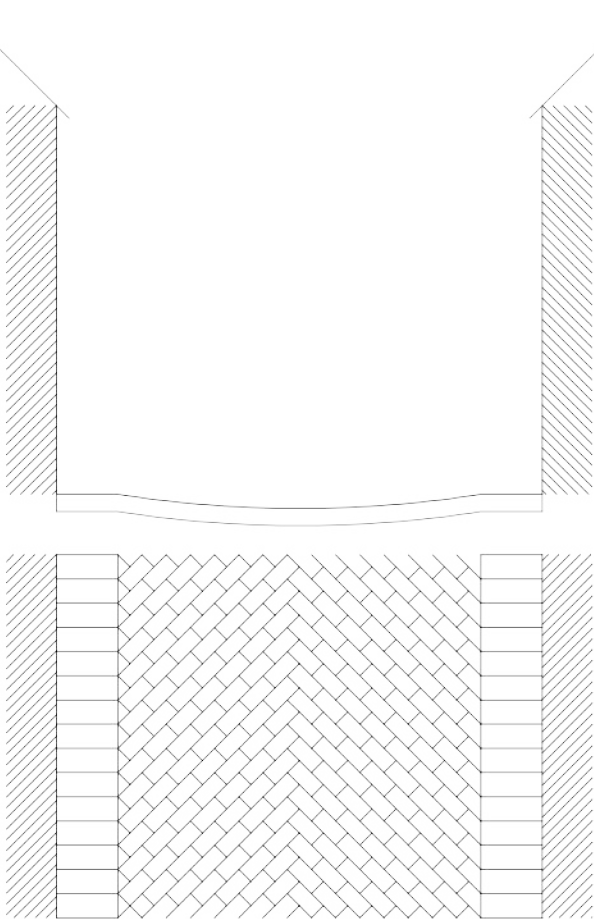
Tipo A5. Conci di pietra con compluvio e disegno centrale a spina di pesce. Ai lati marciapiede a piano stradale con diversa pavimentazione.
