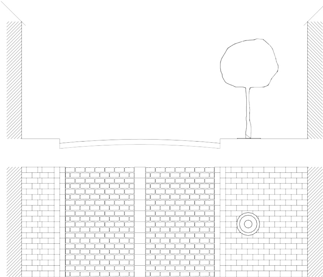
Tipo B5. Basole di pietra a forma irregolare con elemento centrale a basole quadrate. Compluvi laterali in pietra. Marciapiedi in basole di forma regolare.
