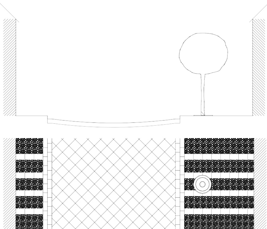
Tipo B4. Basole in pietra di forma quadrata disposte in diagonale. Compluvio centrale. Marciapiede pavimentato con fasce di pietra alternate a ciottoli, presenza di fogliame di medio fusto.
