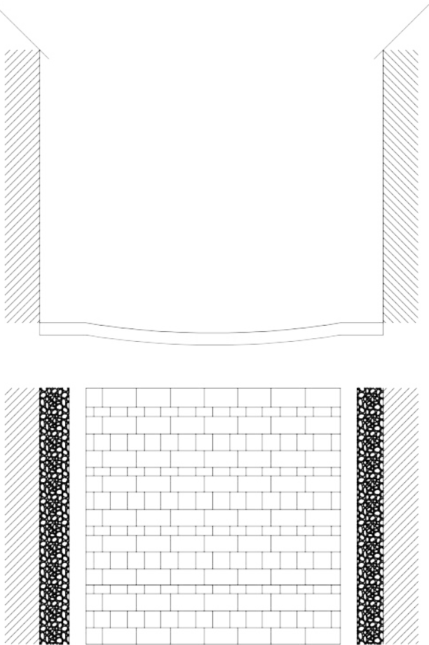
Tipo A2. Mattonelle in pietra disposte a filari di diverse dimensione. Il marciapiede a piano stradale ha una pavimentazione di ciottoli.
