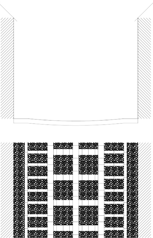
Tipo A3. Riquadri di ciottoli con cornici di pietra. Marciapiede, a piano stradale, pavimentato con ciottoli.
