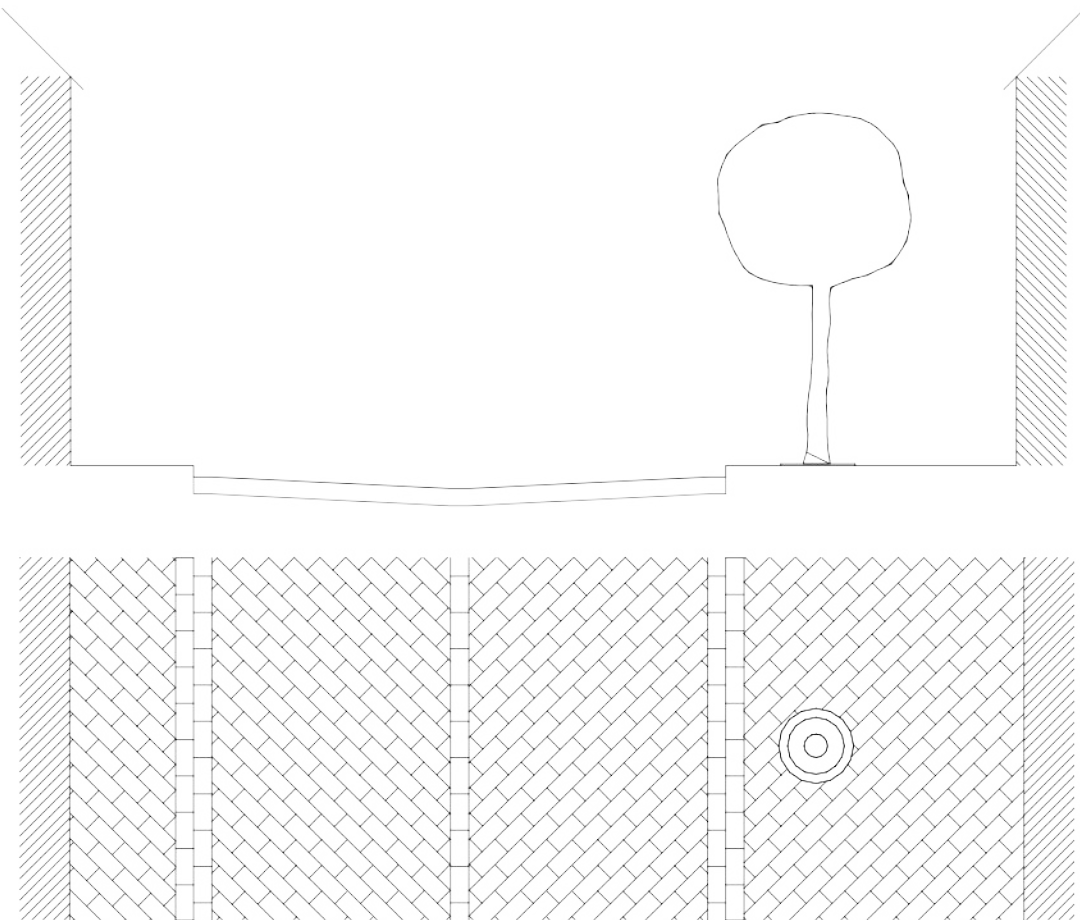
Tipo B1. Basole in pietra con disegno a spina di pesce, compluvio centrale e basole di pietra bocciardate. Marciapiedi con cigli stradali bocciardati e basole in pietra.
