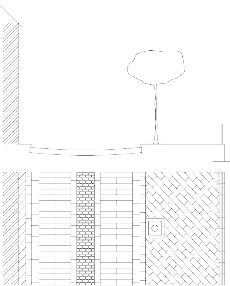
Tipo C4. Basole di pietra di forma regolare, compluvio centrale in conci irregolari. Marciapiedi lastricati con basole in pietra disposte diagonalmente.
