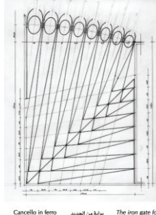
Cancelli in ferro per gli ingressi alla villa بوابة حديدية لمدخل الفيلا The iron gate for the entries to the villa
